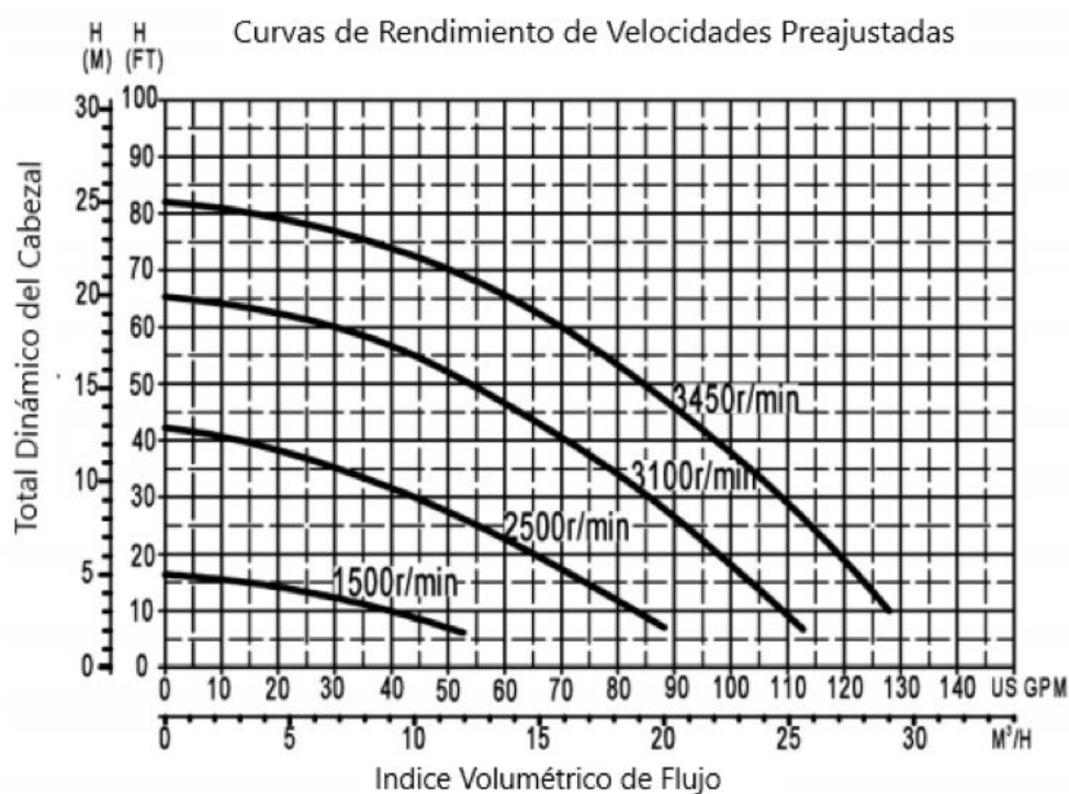
BDXBTVAR200 2.0HP | Curvas de Rendimiento
