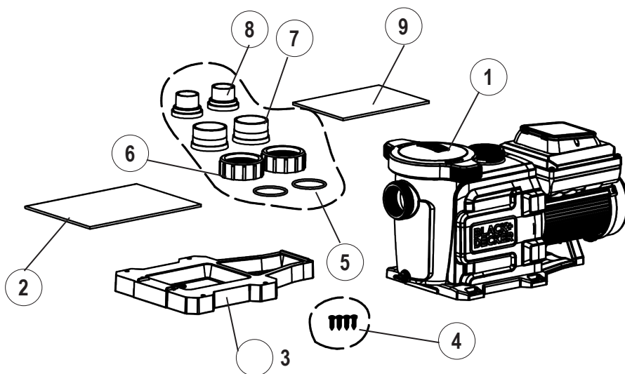
Figure 2. Contenu de l'ensemble de pompes à vitesse variable
